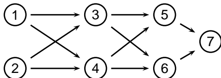
(d) MLP
