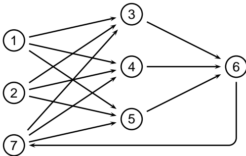
(b) Jordan-Netz mit Kontextneuron
