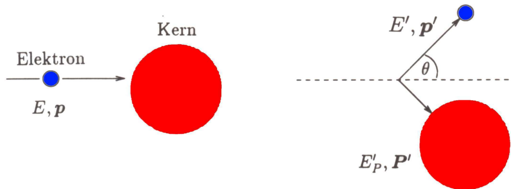
Abb. 5.1. Kinematik der elastischen Elektron-Kern-Streuung
