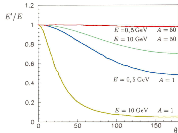
Abb. 5.2. Winkelabhängigkeit der auf die Strahlenergie normierten Elektronstreuenergie E'/E bei elastischer Elektron-Kern-Streuung. Die Kurven zeigen diesen Zusammenhang für zwei verschiedene Strahlenergien (0.5 GeV und 10 GeV) und zwei unterschiedlich schwere Kerne ( A = 1 und A = 50 ).
